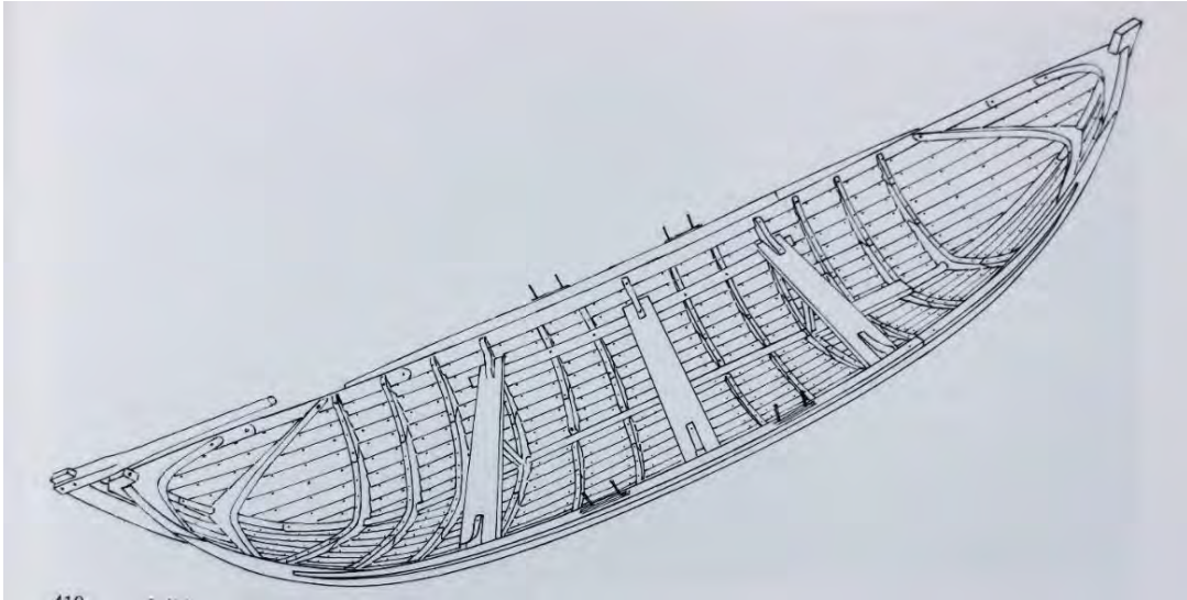
Hindisvíkurbáturinn, yfirlitsteikning. 31
